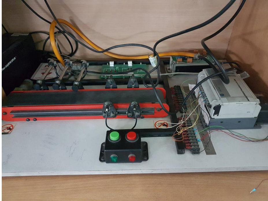
PLC Trainer Kit
